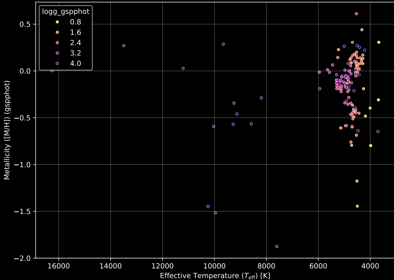
APOGEE DR17 Field: [125-12] Stellar Population Parameters (n= 138)
